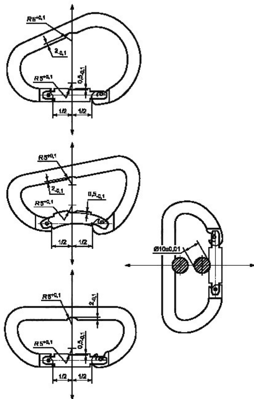
Рисунок 6 — Испытания по малой оси
