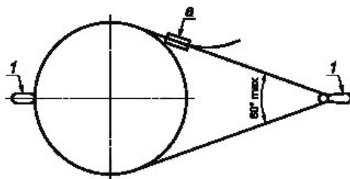
Т — элемент крепления; а — пряжка, которая не должна находиться в контакте с цилиндром
