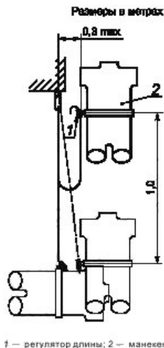
Рисунок 4 — Испытания на динамическую прочность для поясного ремня и строба для рабочего позиционирования
