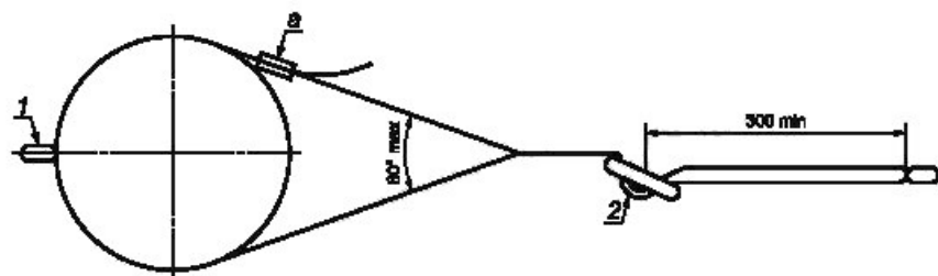
1 — соединительный элемент; 2 — регулятор длины А — пружка, которая не должна находиться в контакте с цилиндром
