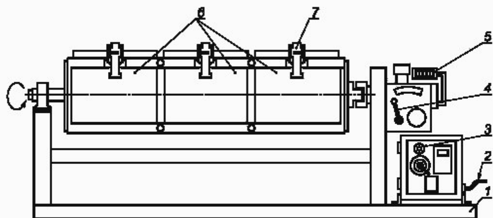
1 — основание; 2 — сетевой шнур; 3 — панель управления; 4 — рычаг узла сцепления; 5 — счетчик; 6 — вращающаяся камера; 7 — металлический затвор
