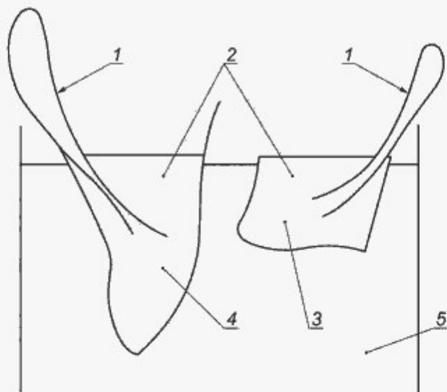
1 — лента, помогающая извлечению формы из испытуемого образца; 2 — оболочки, заправленные воском; 3 — оболочка пяточной части; 4 — оболочка носочной части; 5 — контейнер, заполненный песком
