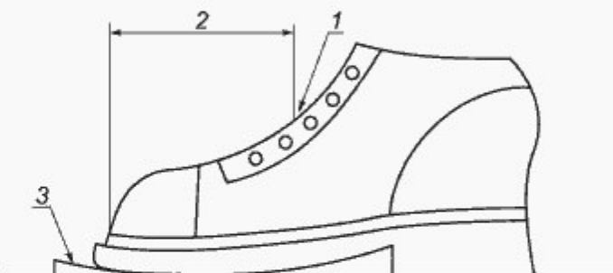
1 — точка удара; 2 — расстояние из таблицы 9; 3 — клин
