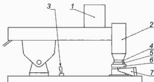
1 — груз; 2 — установленные в корпус нагревательные блоки, включающие устройство измерения температуры; 3 — вил/выкл тумблер; 4 — квадратный конец медного бита; 5 — испытуемую пробу; 6 — самовыравнивающаяся платформа для испытуемого образца; 7 — шарнирная теплоизолированная опора
