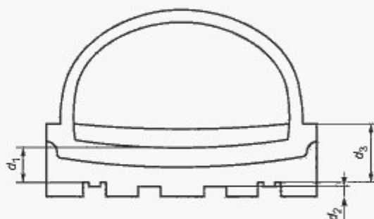
Рисунок 29 — Резиновая и полимерная обувь (протектор)
