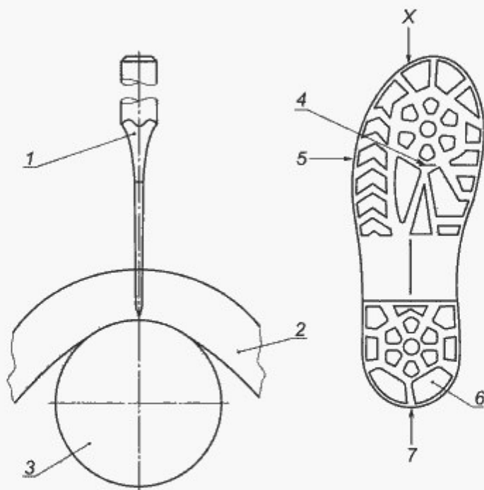
1 — режущий инструмент; 2 — испытуемая проба; 3 — ролик испытательной машины, радиусом 15 мм; 4 — линия разреза подошвы, параллельная АС ; 5 — линия АС (линия сгибания подошвы); 6 — протекторы (шины); 7 — продольная ось XY
