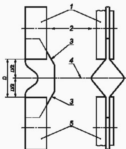
1 — неподвижные зажимы; 2 — центр направляющих штифтов диаметром приблизительно 6 мм; 3 — клиновидные козлы испытуемого образца; 4 — центральная ось испытуемого образца; 5 — зажим, совершающий возвратно-поступательное движение
