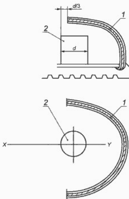
Рисунок 6 — Положение цилиндра при испытании на удар и сжатие
