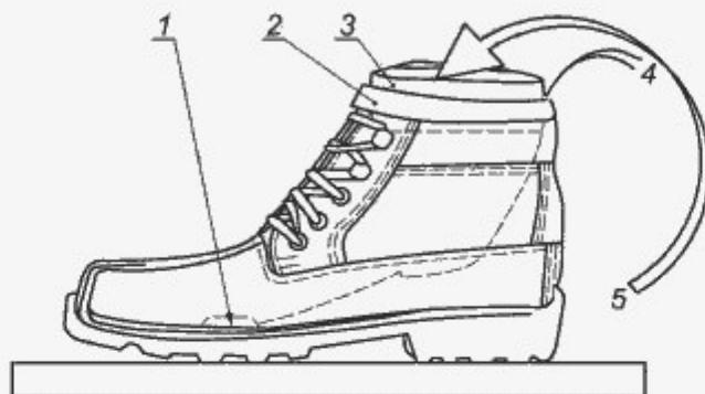
1 — точка измерения температуры; 2 — ленты соединения верха обуви с удлиняющим рукавом; 3 — заглушка; 4 — провода к термодатаре; 5 — стальные шарики (здесь не показаны)
