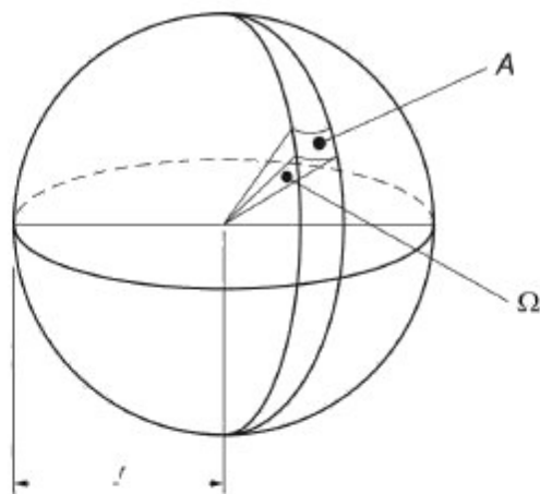
\Omega — телесный угол в стерadians ( \Omega = A/r^2 ); A — площадь поверхности на воображаемой сфере; r — радиус воображаемой сферы
