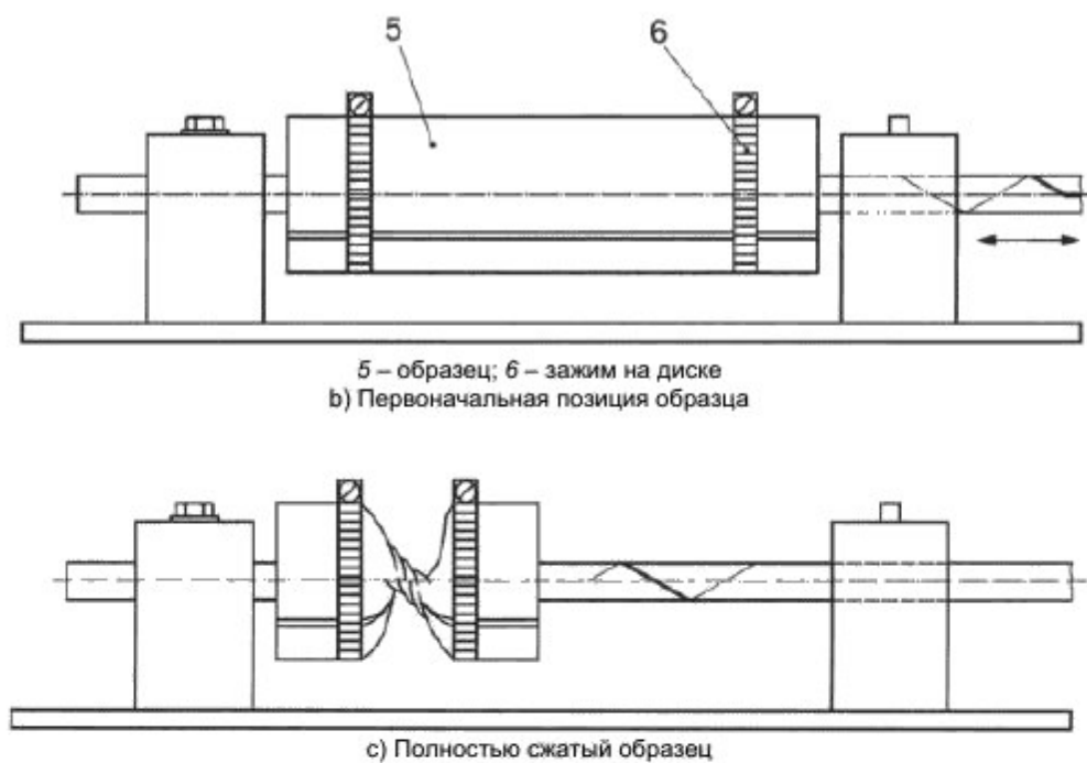
Рисунок А.1 - Испытательная установка для механической подготовки образцов
