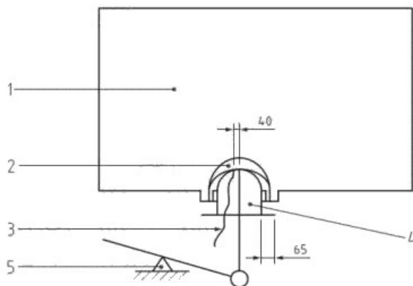
1 – термокамера; 2 – испытуемый образец; 3 – термопара; 4 – термомакет; 5 – подъемное устройство
