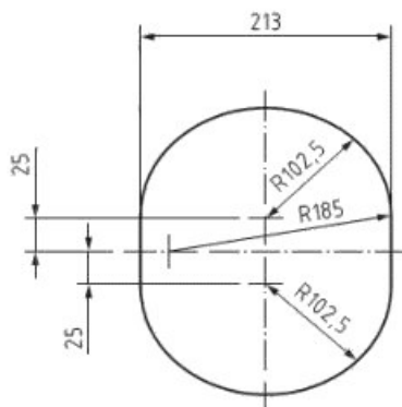
Рисунок 2 — Размеры отверстия в нижней части термокамеры
