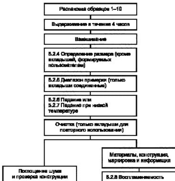
Рисунок В.3 — Блок-схема испытания вкладышей
