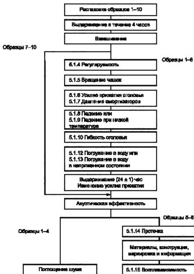
Рисунок В.1 — Блок-схема испытаний наушников с оголовьем
