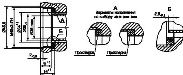
Рисунок Б.4 — Резбовое соединение с внутренней резьбой для систем с двумя каналами подачи воздуха PIB
