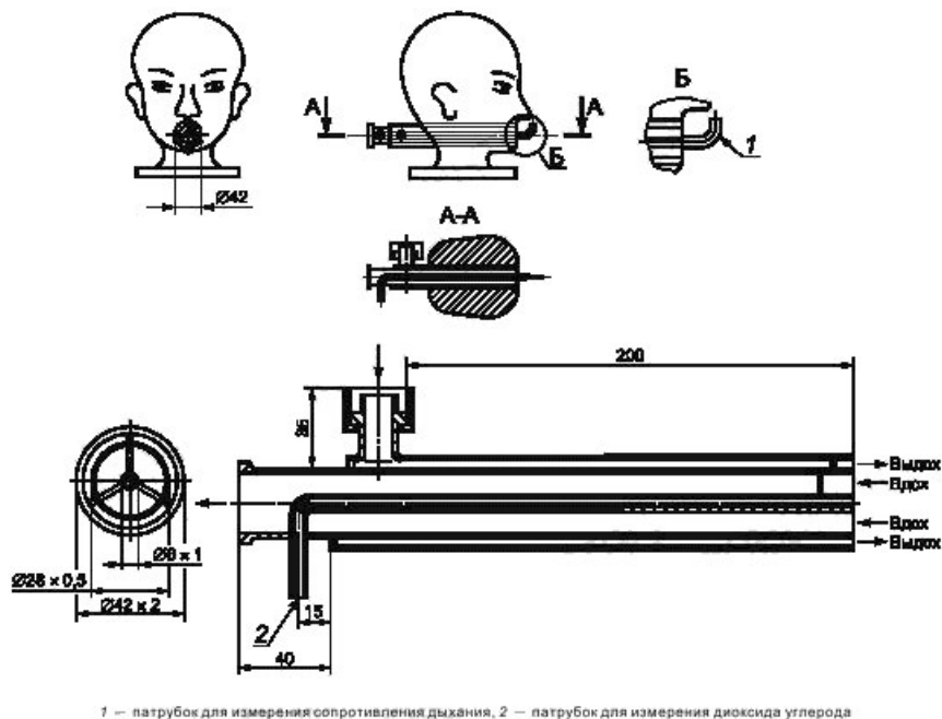
Рисунок 3 — Муляж головы человека (голова «Шеффилда»)
