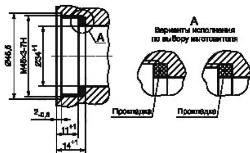
Рисунок Б.3 — Резбовое соединение с внутренней резьбой для систем с одним каналом подачи воздуха PIA
