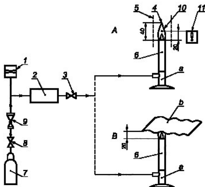
А — измерение температуры пламени; В — испытание образца материала 1 — манометр, 2 — предохранительный клапан, 3 — устройство регулирования давления; 4 — пламя, 5 — экран; 6 — горелка, 7 — баллон с пропаном; 8 — вентиль; 9 — регулятор давления; 10 — термометр; 11 — устройство измерения температуры. а — воздушный клапан закрыт; б — испытываемый материал
