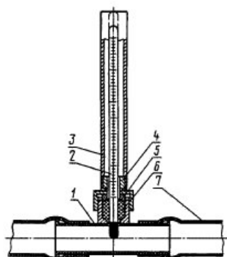
Схема установки термометра в линию
