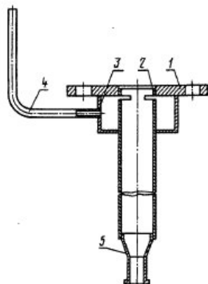
Схема входного штуцера
