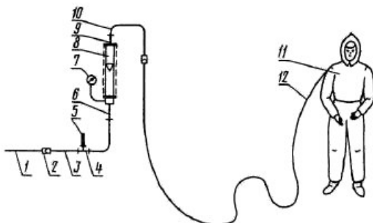
Схема установки ротаметра в технологическую линию
