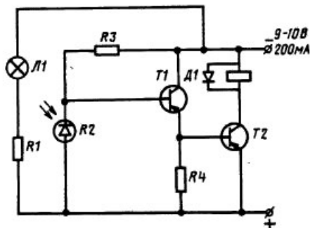
Электрическая схема автоматического датчика
