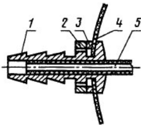
Схема крепления штуцера к СИЗ ОД
