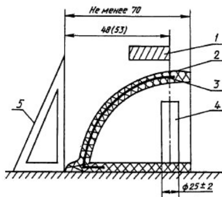
1 — боек; 2 — носок; 3 — ударозащитный подносик; 4 — пластилиновый столбик; 5 — угольник
