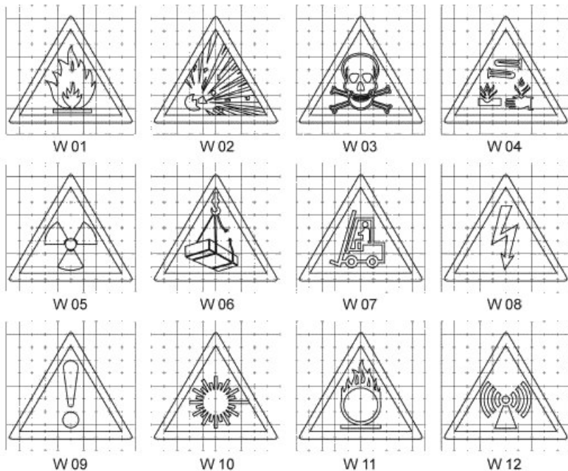
Рисунок П.2, лист 1 — Предупреждающие знаки
