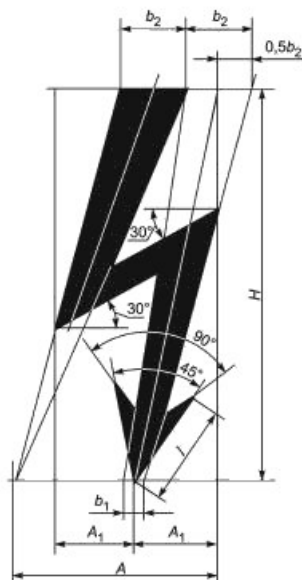
Рисунок Н.1 — Графический символ электрического напряжения
