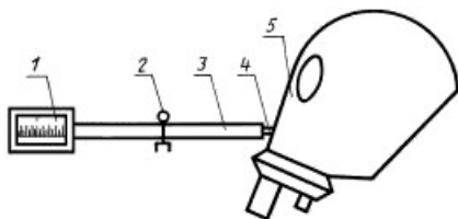
1 — прибор для измерения избыточного давления и разрежения под лицевой частью СИЗОД; 2 — зажим; 3 — трубка резинового вентиля; 4 — штуцер; 5 — СИЗОД (условно показана только лицевая часть)
