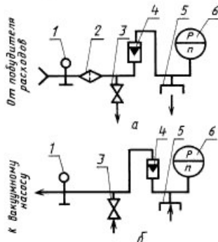
а — режим «выдох», б — режим «вдох». 1 — зажим; 2 — фильтр; 3 — регулировочный вентиль; 4 — ротаметр; 5 — насадка для подключения устройства, герметизирующего лицевую часть; 6 — титаноломер
