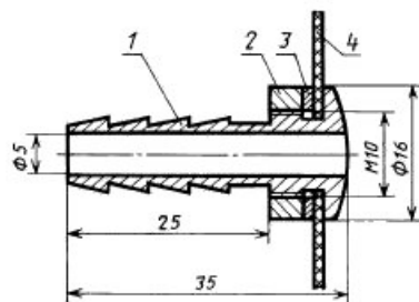
1 — штуцер; 2 — гайка; 3 — шайба; 4 — лицевая часть СИЗОД Черт. 1
