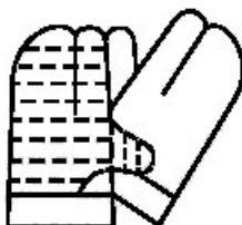
Рисунок А.2 — Перчатка трехпалая
